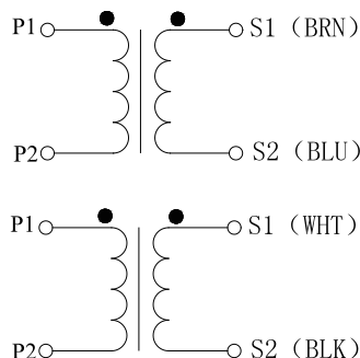
原理图
